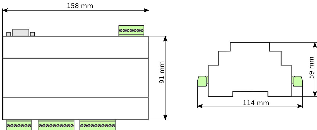
Fig. 4. RB100-CM3 dimensions
