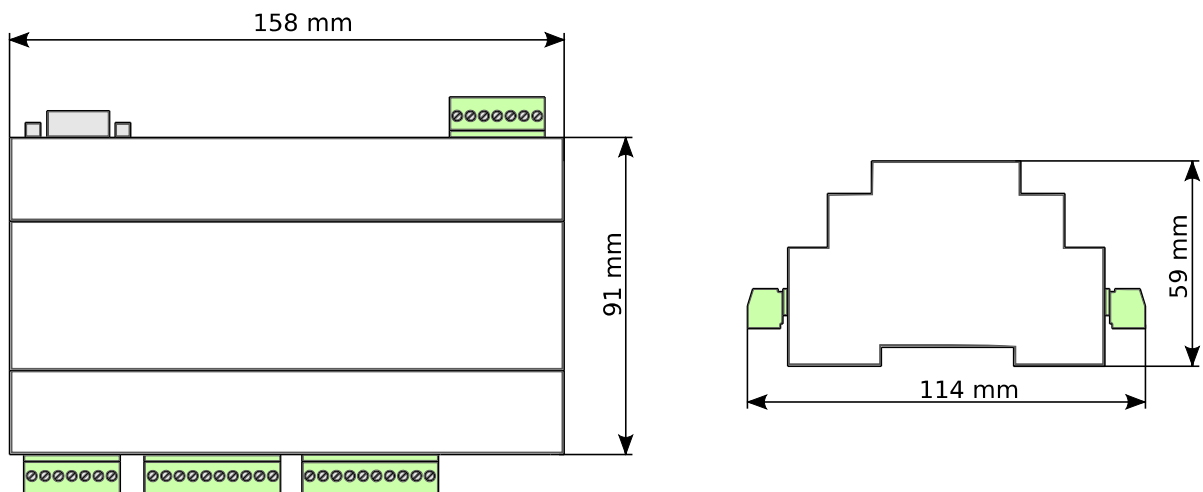
Fig. 4. RB100-CM3 dimensions
